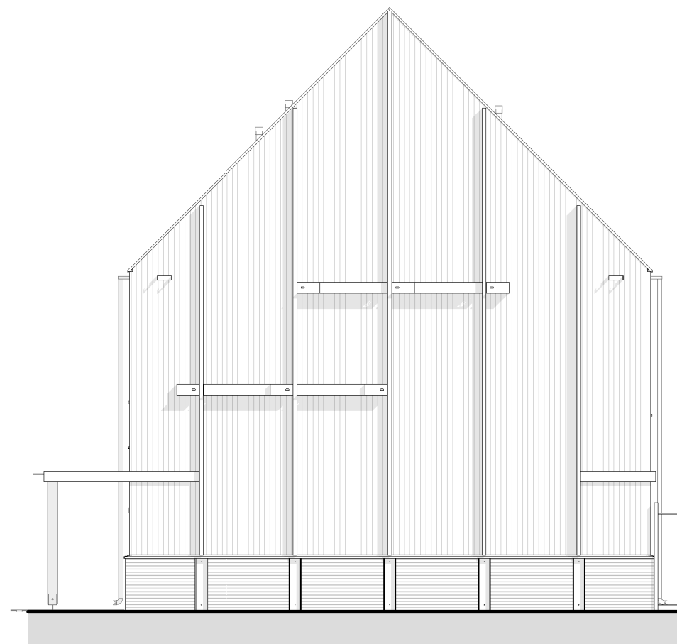
kopgevel met huiszwaluw nestkasten bnr. 51 (noord)
