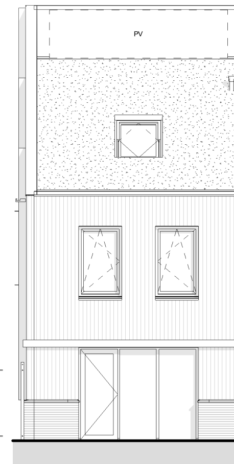
achtergevel (west)
