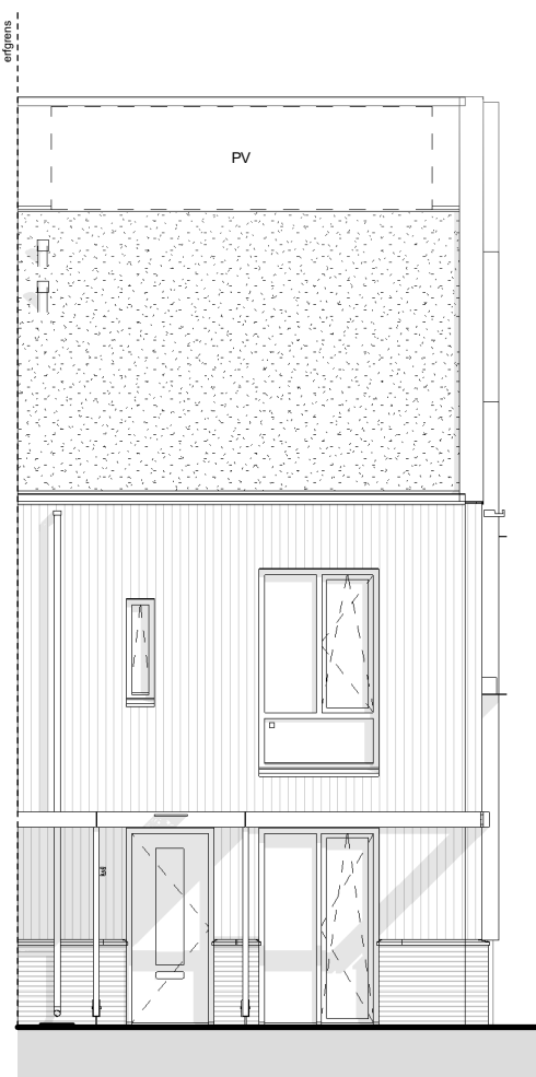
voorgevel (oost)
