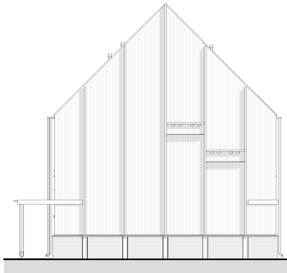
kopgevel met gierzwaluw nestkasten bnr. 58 (noord)
